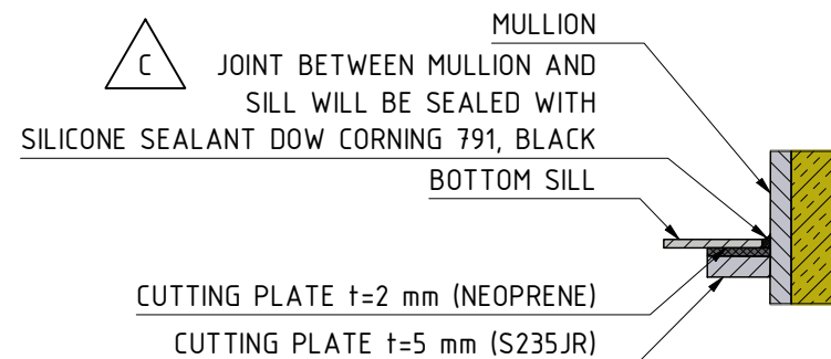
SECTION Y-Y (1 : 2)
