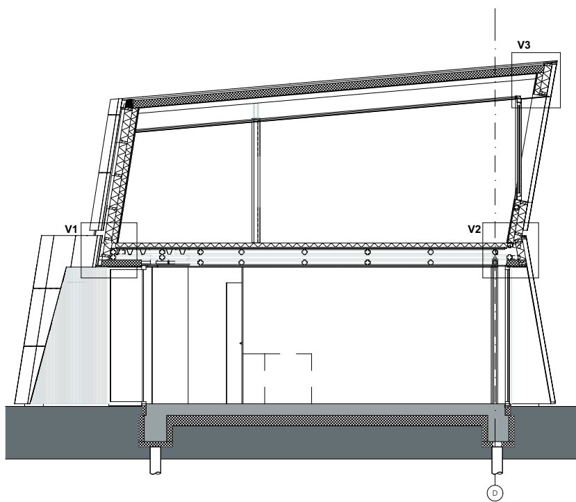
Doorsnede B-B
