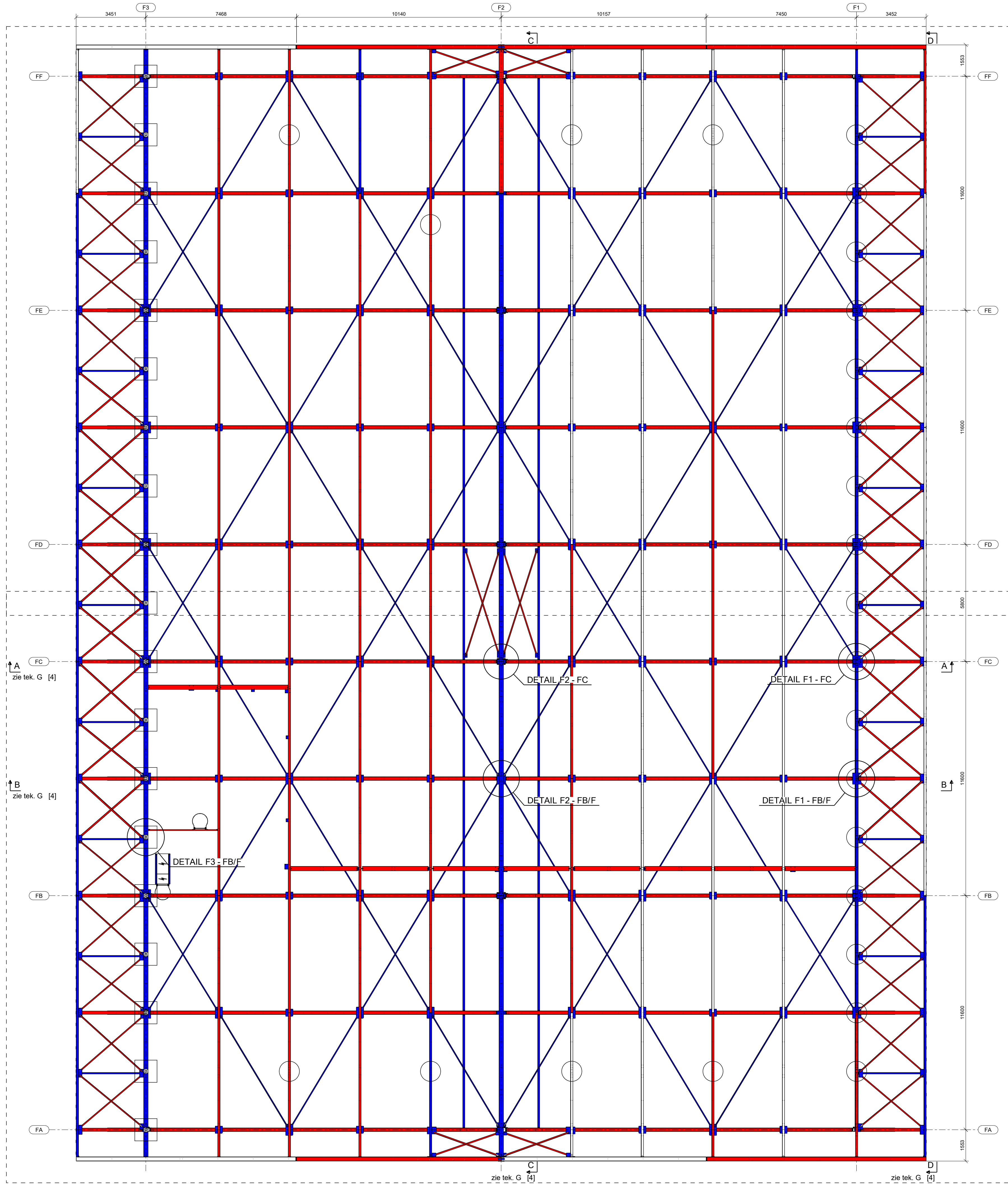
Bovenaanzicht, 1:105
