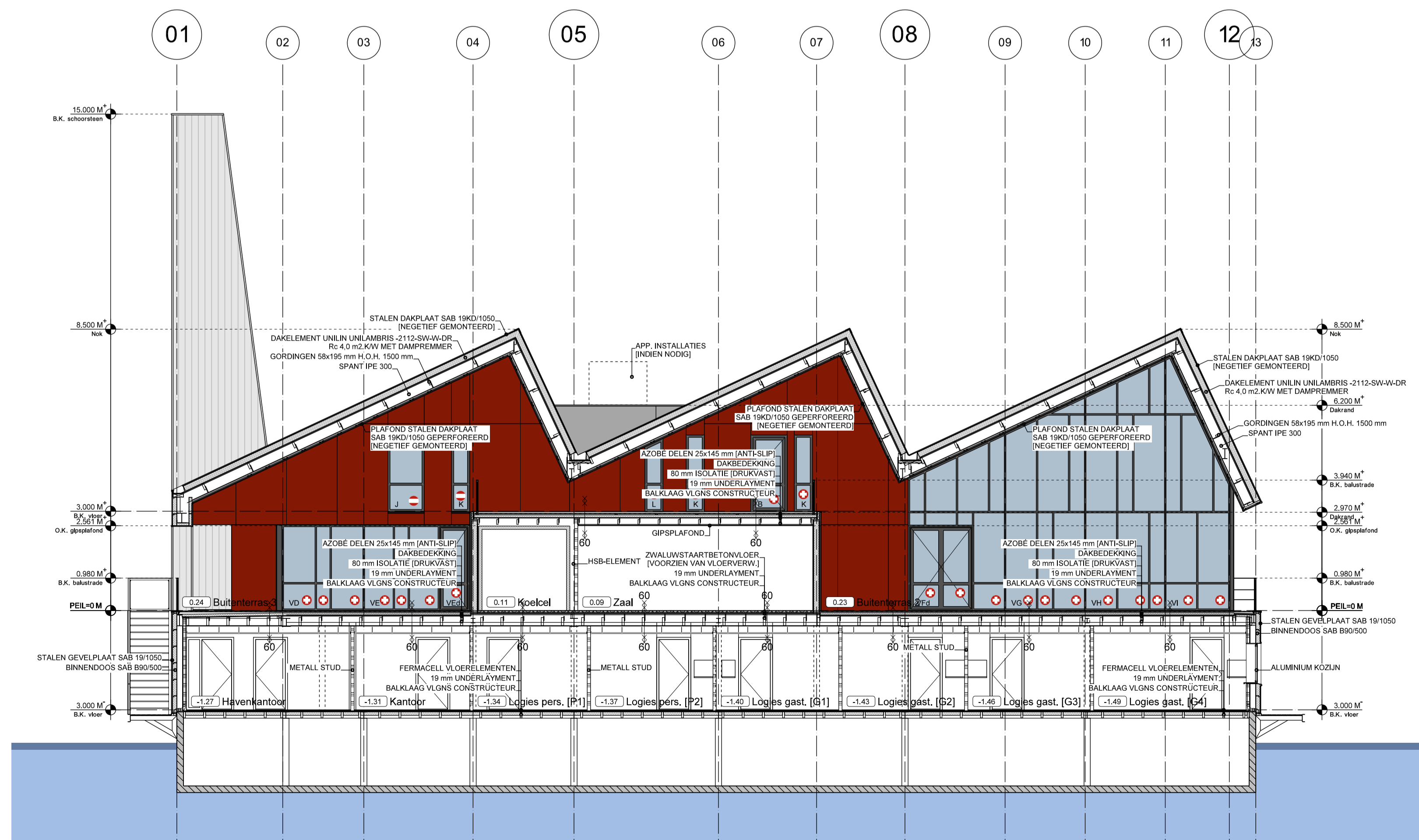
DOORSNEDE C - C
