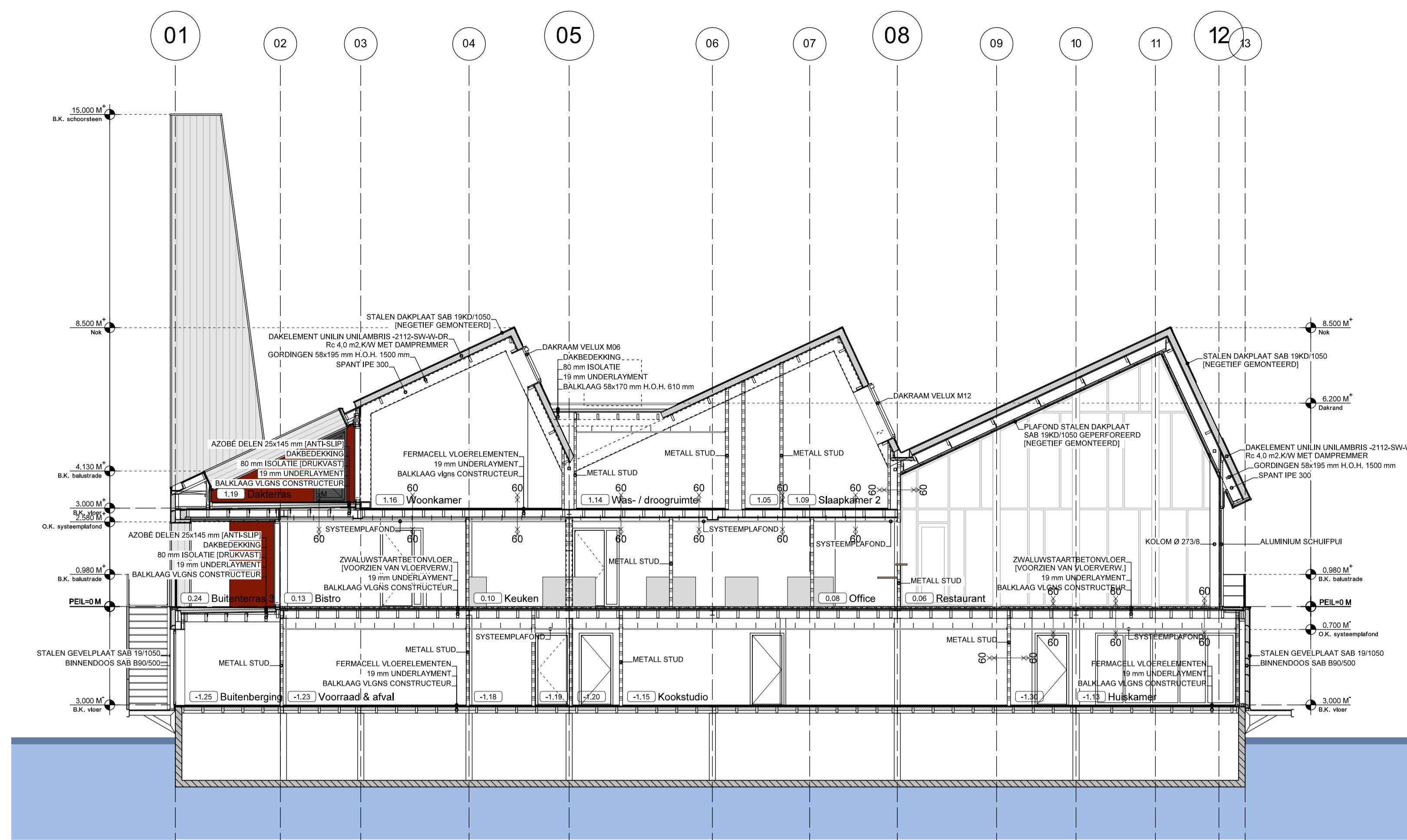
DOORSNEDE A - A
