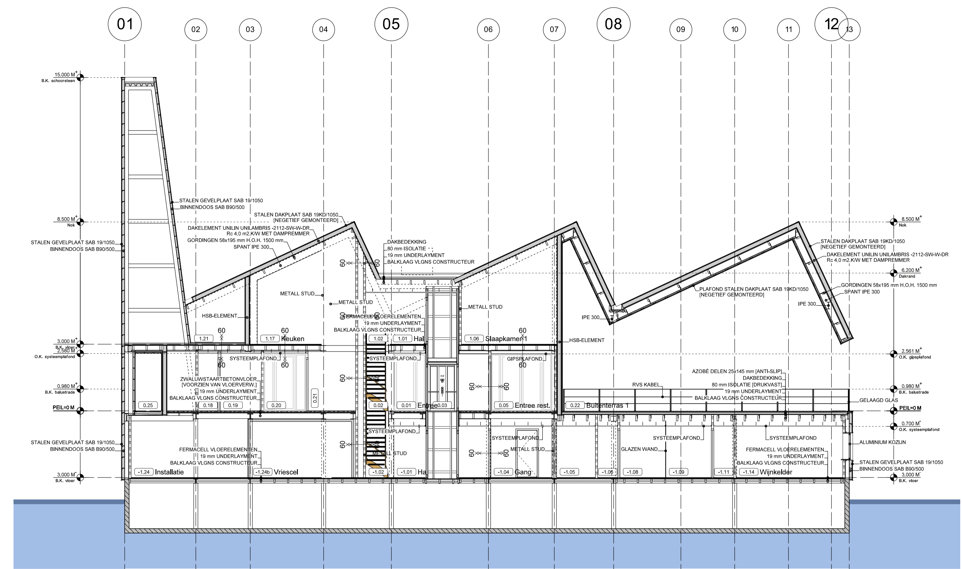
DOORSNEDE B - B
