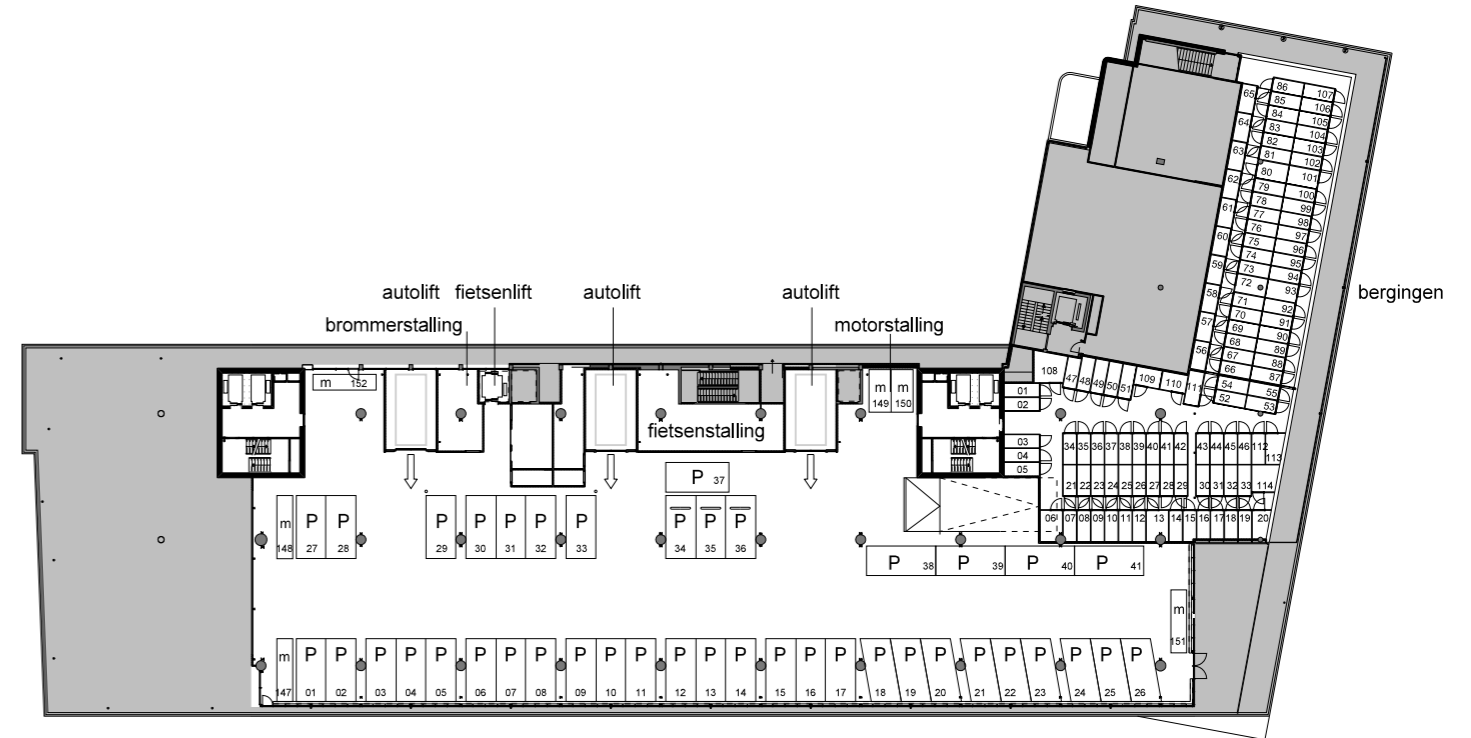
4e verdieping parkeren auto's fietsen brommers en bergingen appartementen
