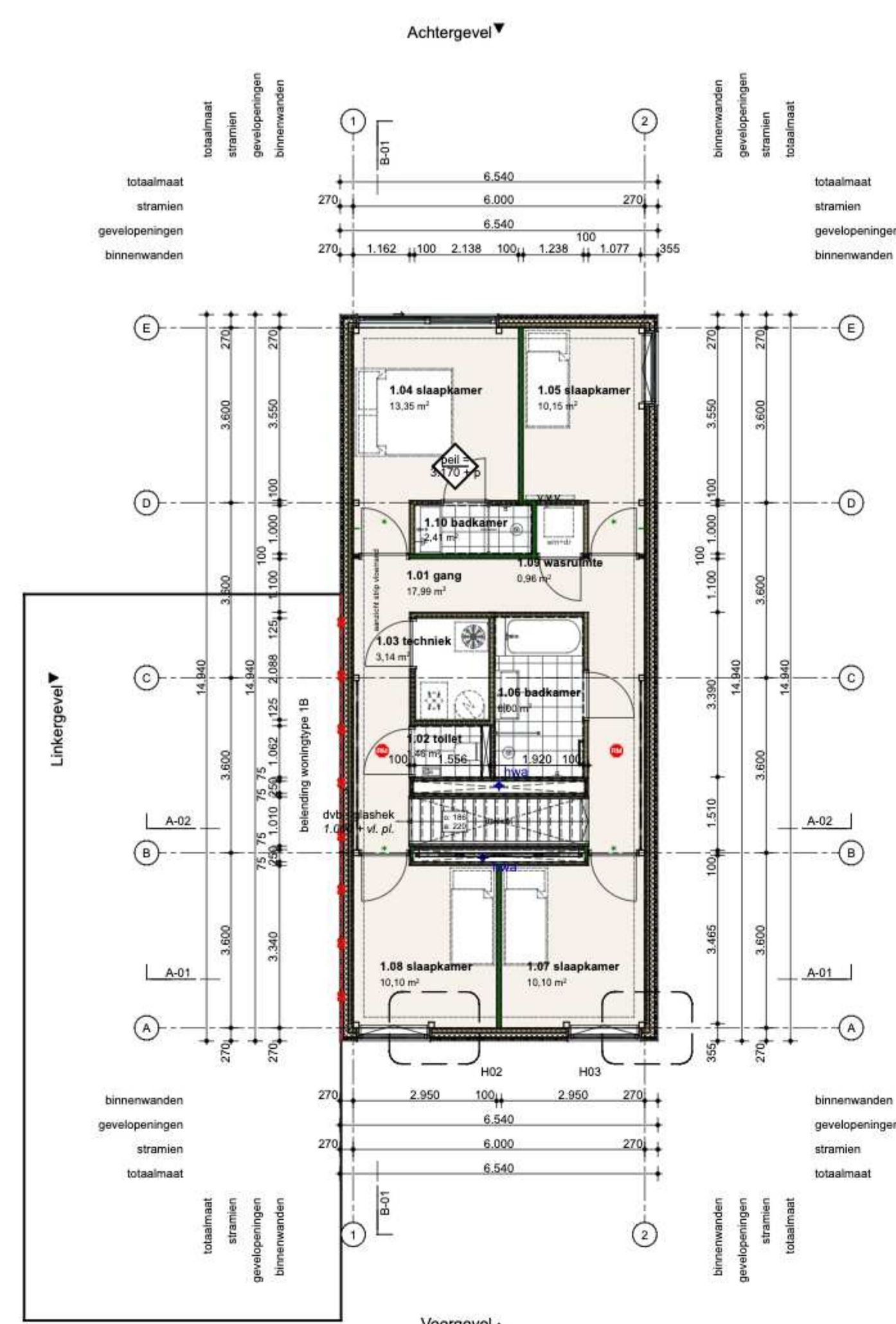
01a eerste verdieping
