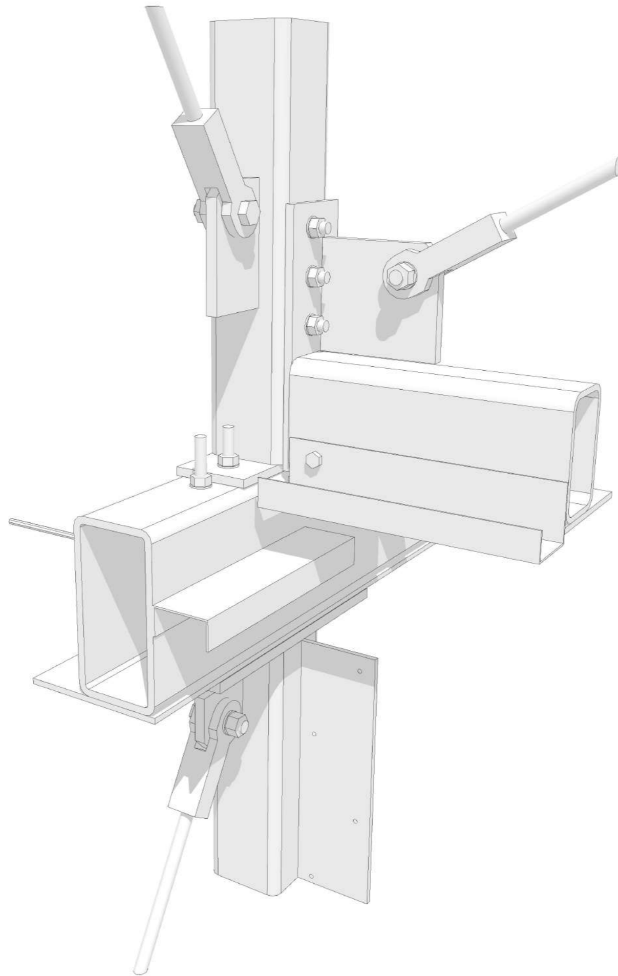
staalknooppunt
