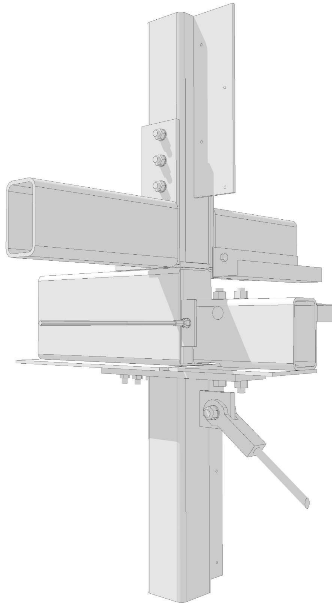
staalknooppunt
