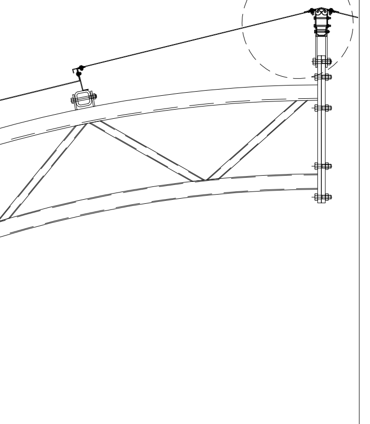
Coupe: principe zone tôle métallique
