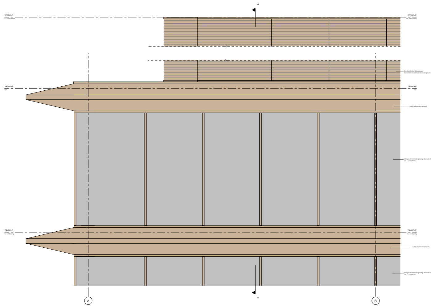
Aanzicht 1:20
