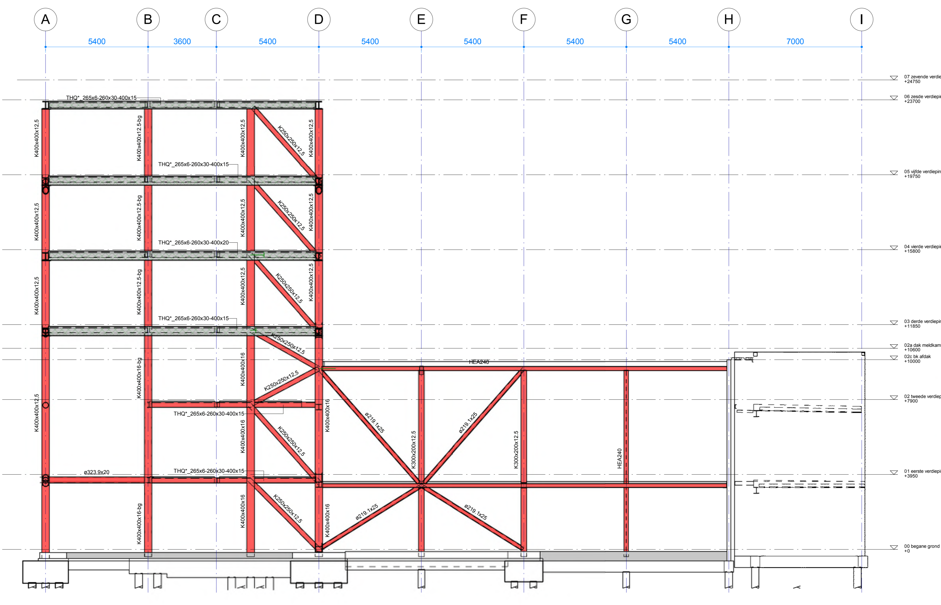
Wandaanzicht G-9 Schaal: 1 : 100
