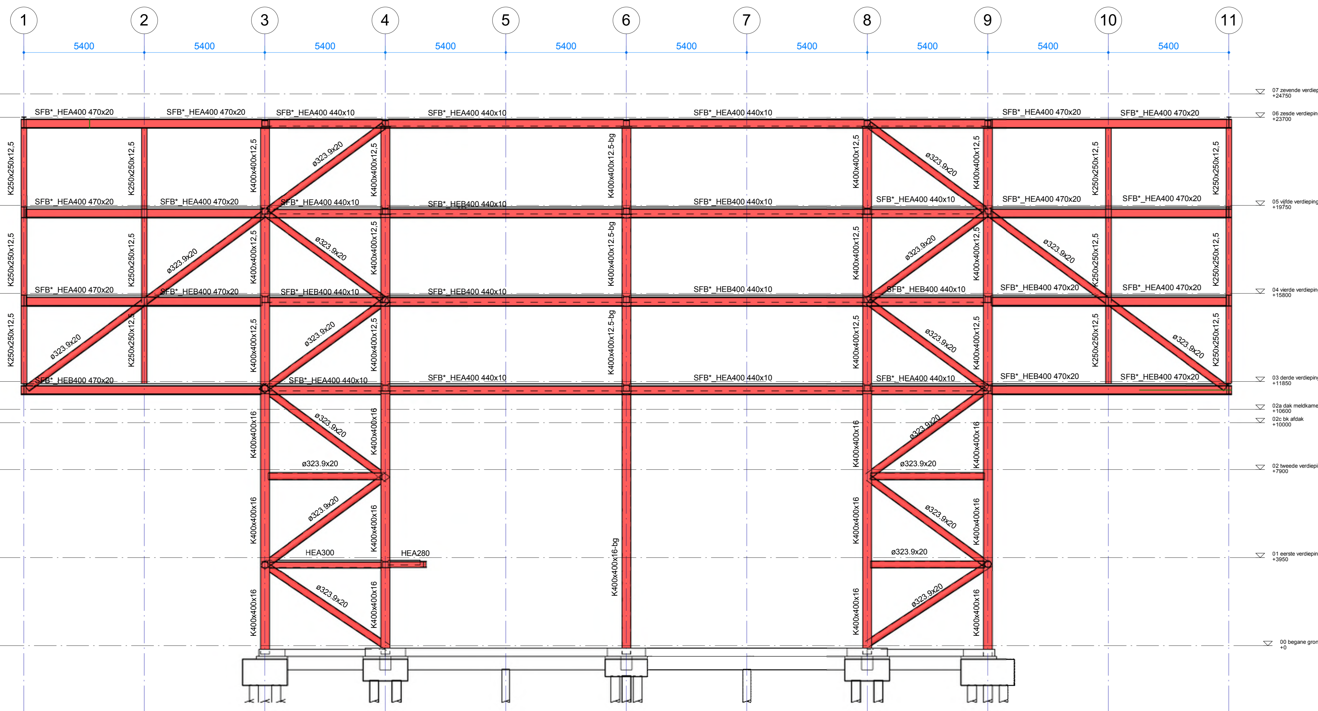
Wandaanzicht G-A Schaal: 1 : 100
