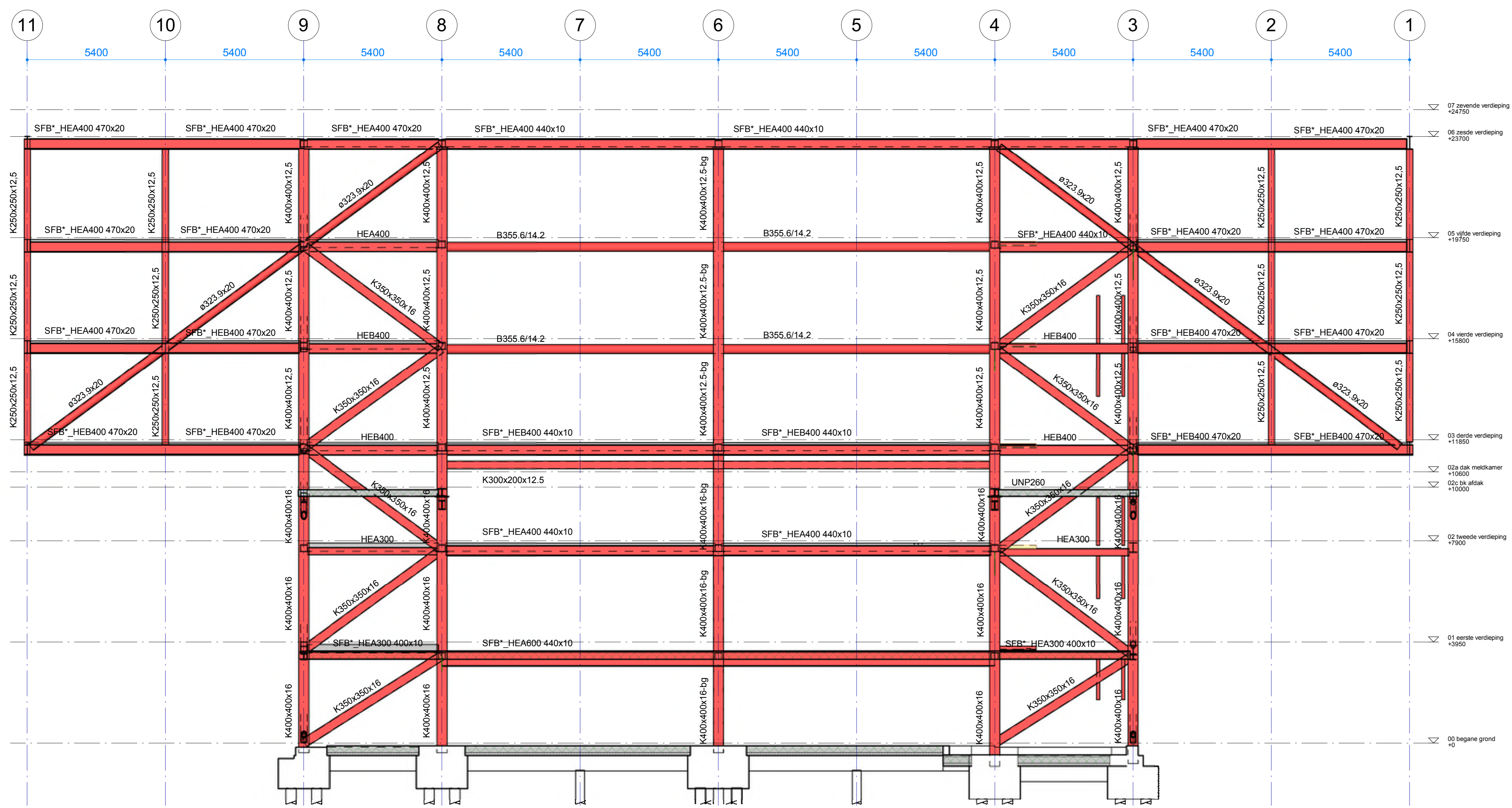
Wandaanzicht G-D Schaal: 1 : 100
