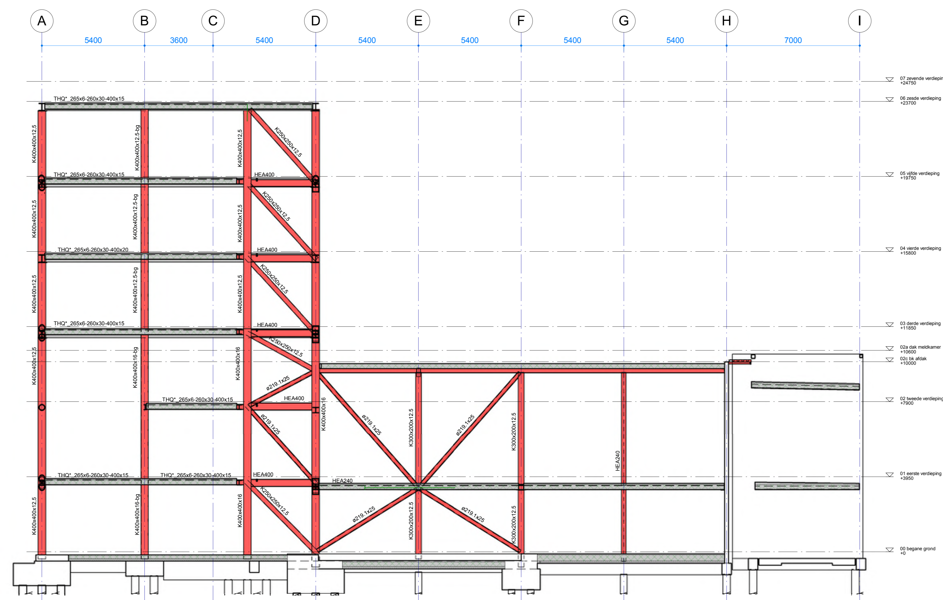
Wandaanzicht G-3 Schaal: 1 : 100
